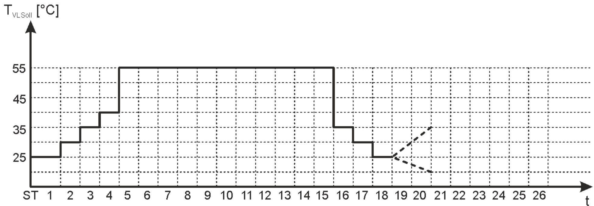
Abb. 49: Zeitlicher Ablauf - Belegreifheizen
