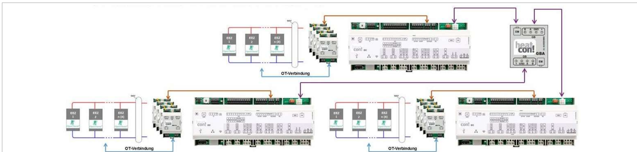
Abb. 36: OpenTherm Kaskade Vollausbau
