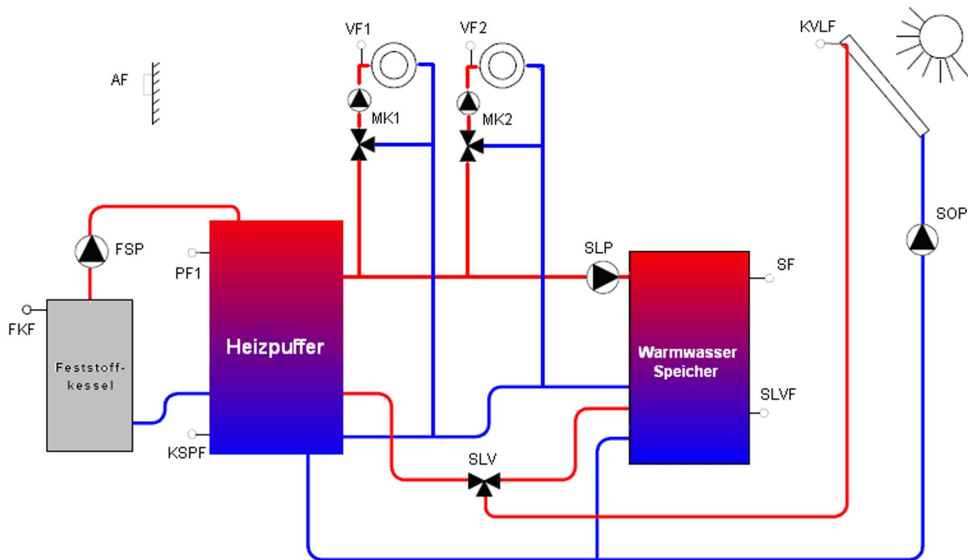
Abb. 54: Feststoffregelung mit Solar und Solarladeventil
