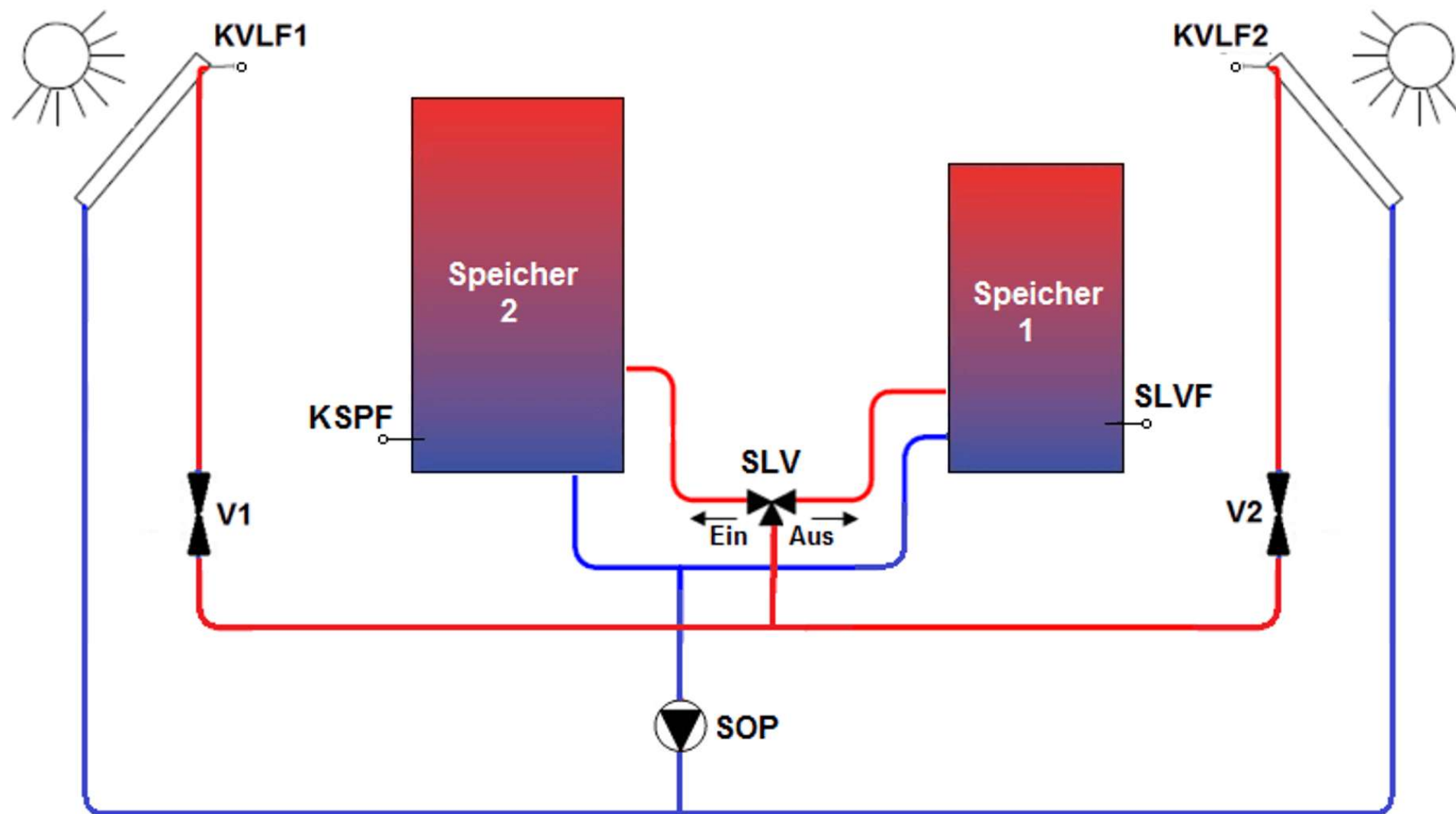
Abb. 63: Doppel-Kollektoranlage und Doppelpuffersystem mit Ladeventilumschaltung
