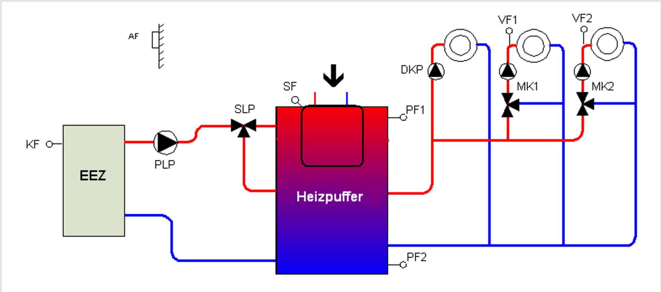
Abb. 57: Pufferladeregelung mit Warmwasserumlenkventil
