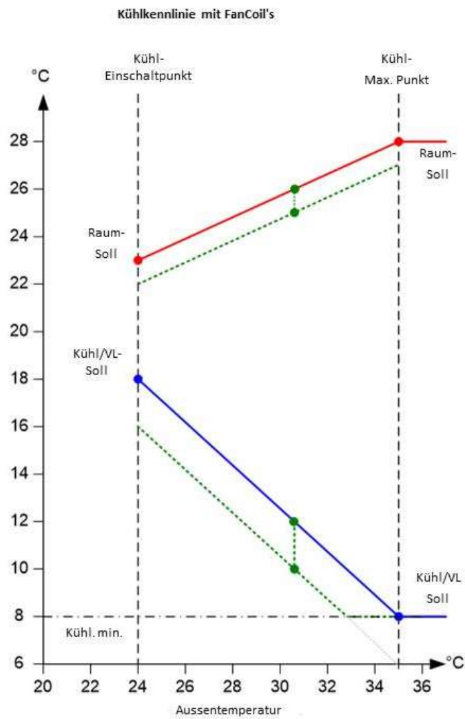
Abb. 42: Zusammenhang Raum-Solltemperatur ⇔ Vorlauftemperatur
