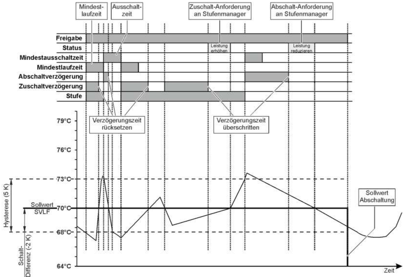
Abb. 32: Stufenmanager (Beispiel)
