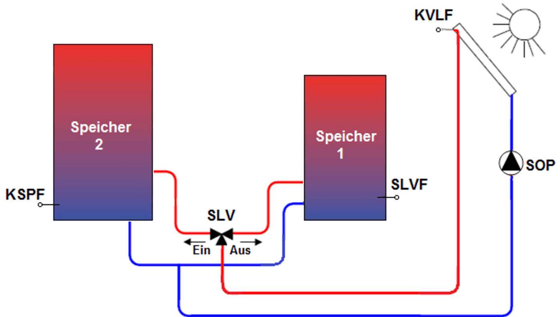
Abb. 61: Doppel-Puffersystem einer Solaranlage (Beispiel)
