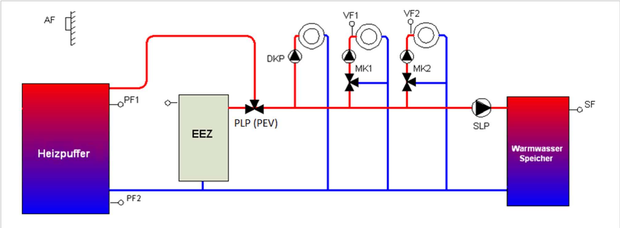
Abb. 58: Pufferentladeregelung auf HK und WW
