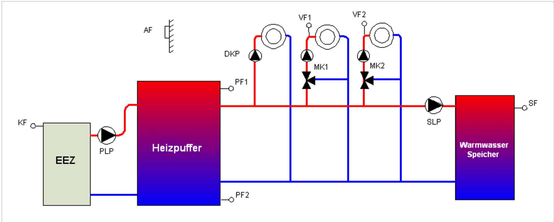
Abb. 53: Pufferladeregelung mit Heizkreis- und Warmwasseranforderung
