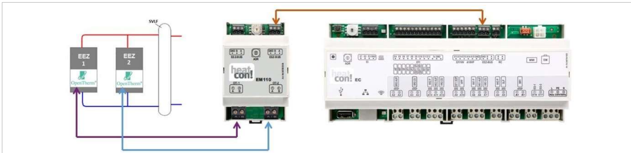
Abb. 35: OpenTherm Kaskade
