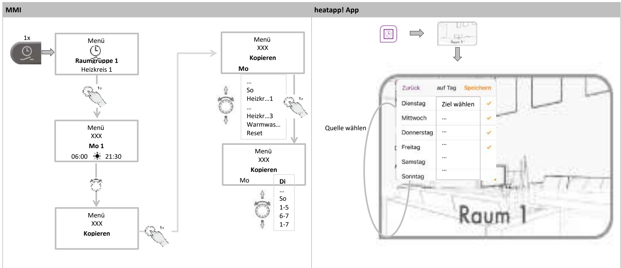
Abb. 23: Schaltzeiten kopieren
