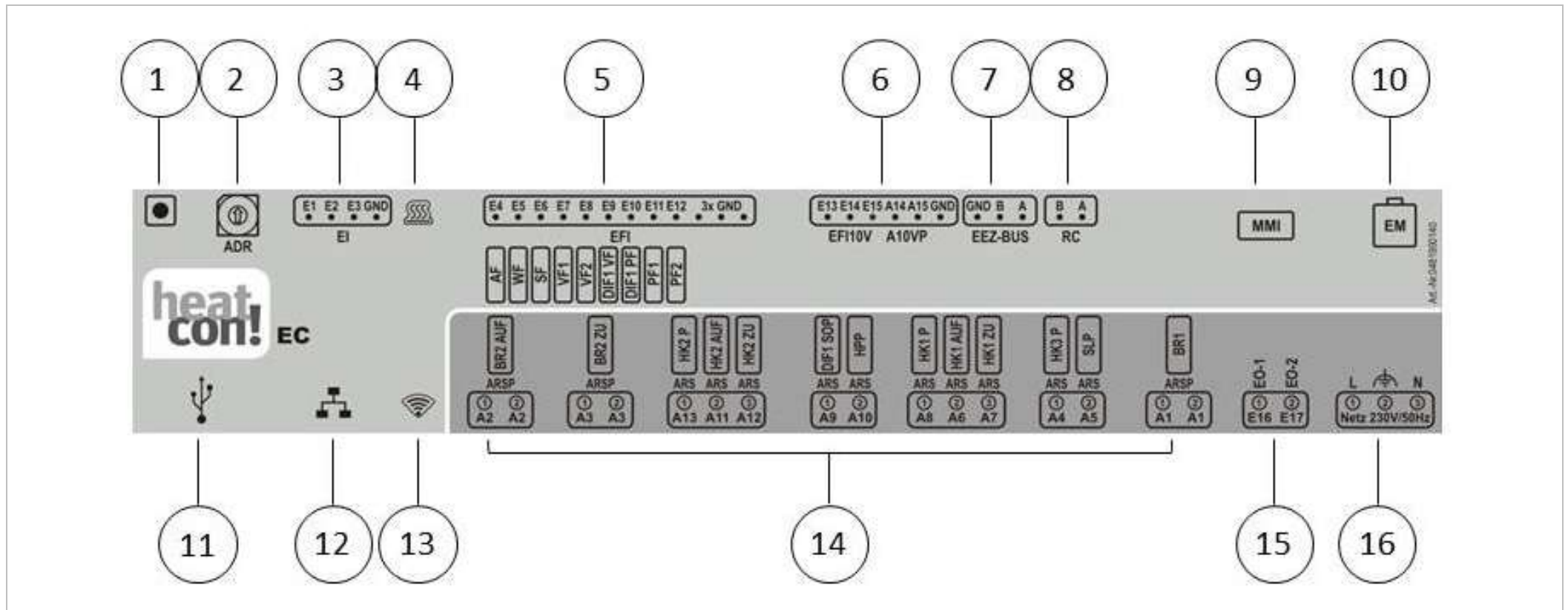
Abb. 28: heatcon! EC – Anschlussbelegung
