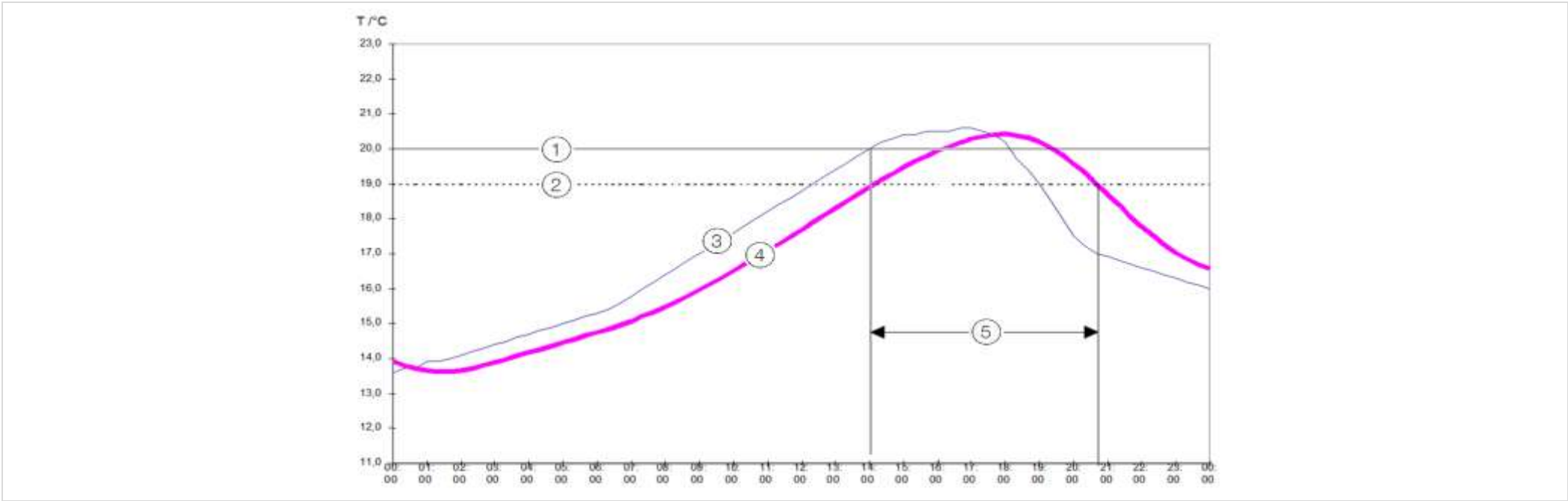
Abb. 46: Sommerbetrieb
