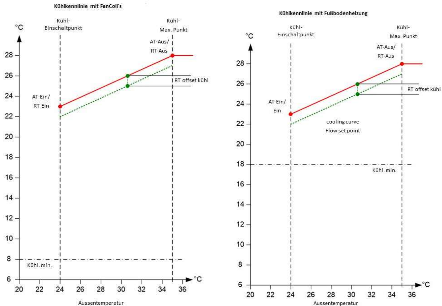
Abb. 41: Ermittlung Raum-Solltemperatur
