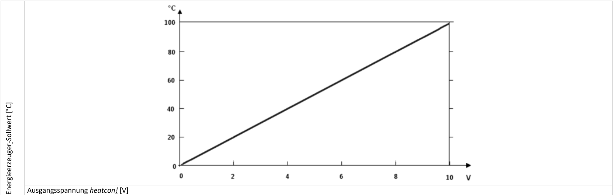
Abb. 33: Kennfeld ohne Anpassung an den Energieerzeuger
