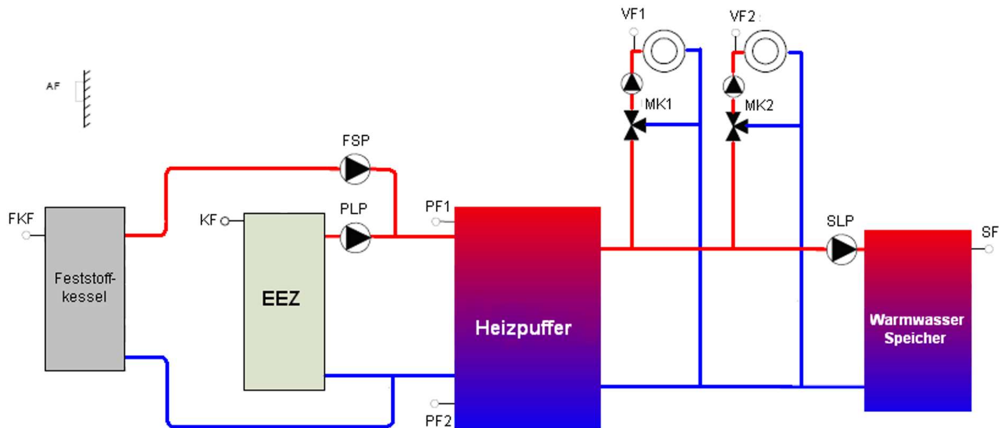
Abb. 55: Pufferladeregelung mit Feststoffkessel für HK und WW
