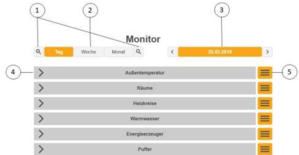
Abb. 13: Monitor Startseite
