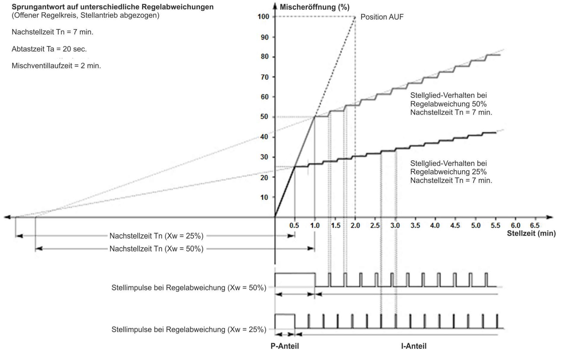
Abb. 39: Beispiel für das Zusammenwirken der Regelparameter
