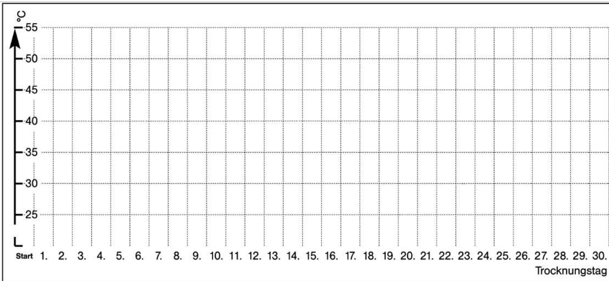
Abb. 51: Zeitlicher Ablauf manuelle Einstellung Estrich Funktion
