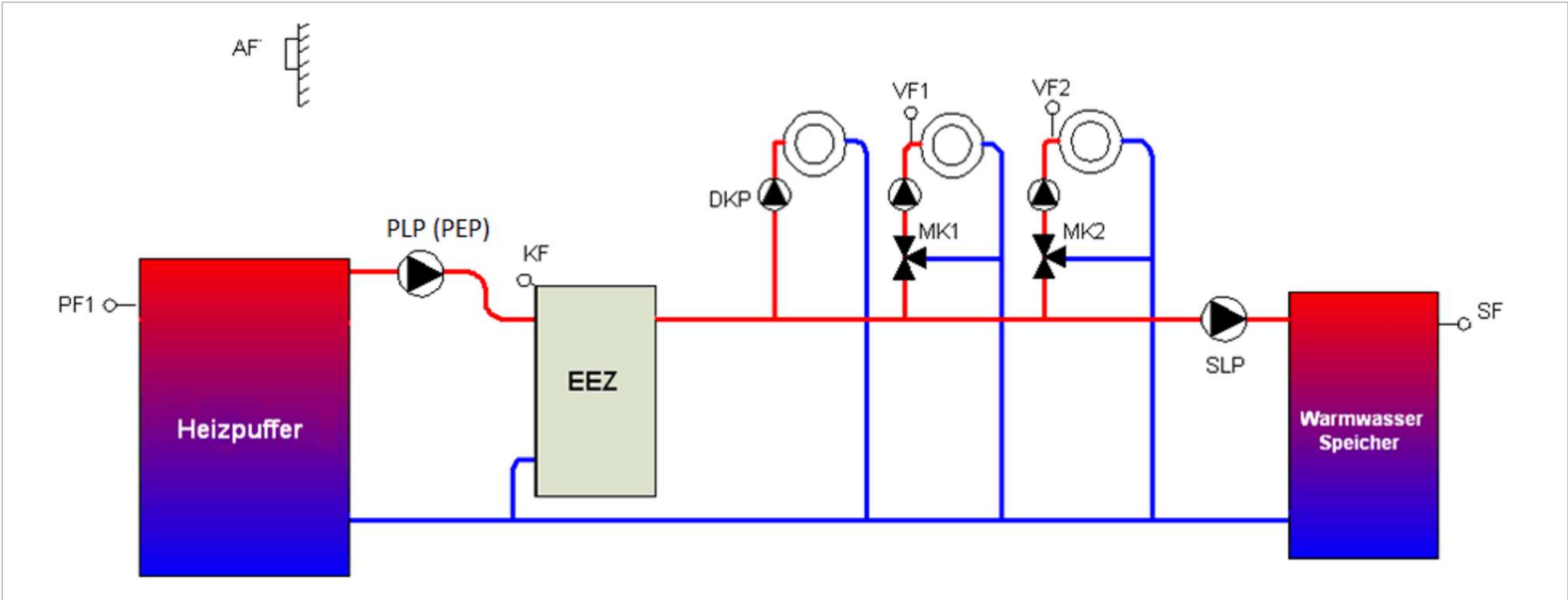
Abb. 60: Pufferentladeregelung 2 auf Wärmeerzeuger
