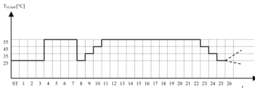
Abb. 72: Zeitlicher Ablauf - Funktionsheizen mit nachfolgendem Belegreifheizen
