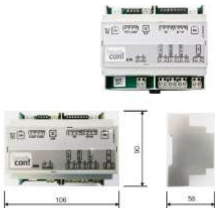
heatcon! Erweiterungsmodul EM 100
