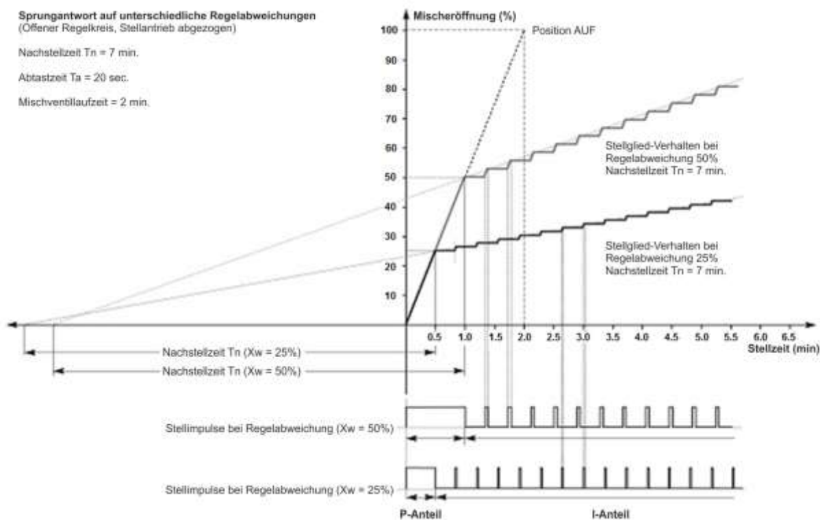
Abb. 61: Beispiel für das Zusammenwirken der Regelparameter
