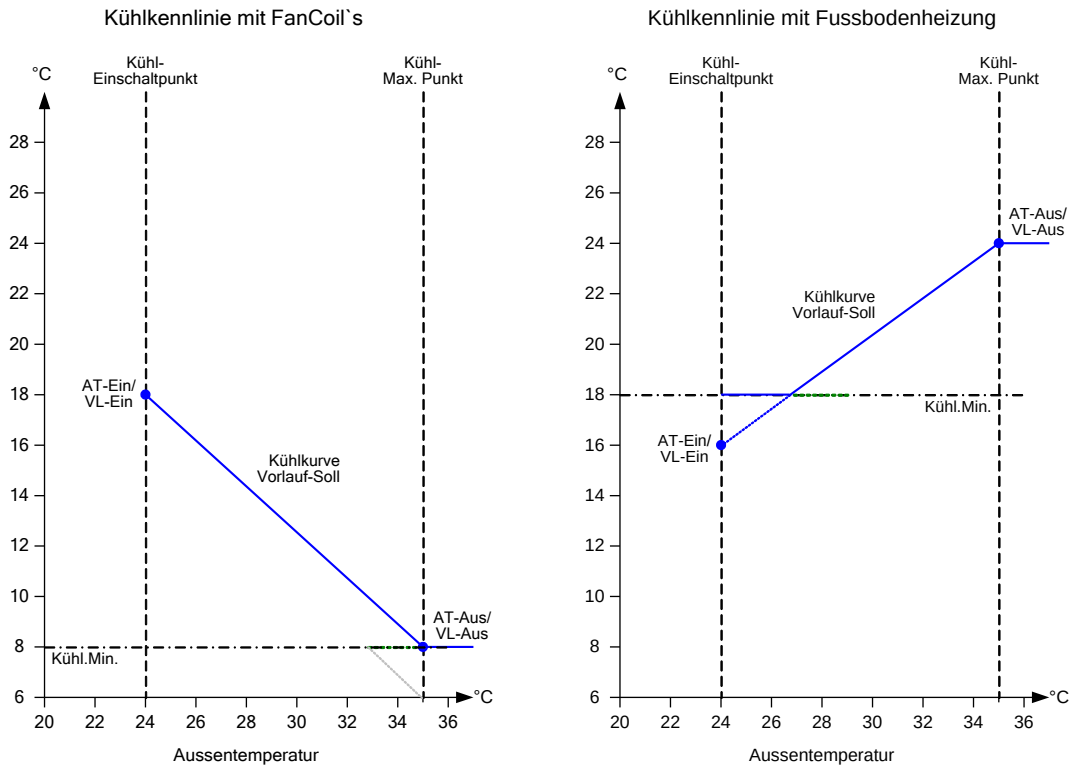
Abb. 62: Kühl-Kurve
