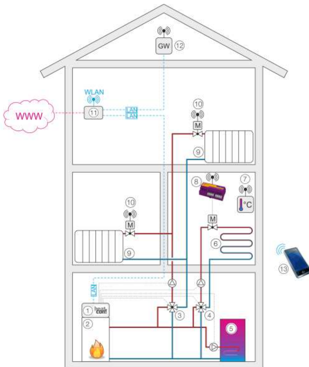
Abb. 1: Systemübersicht (Beispiel)
