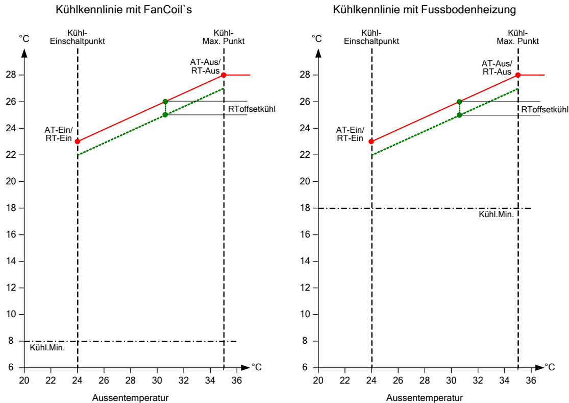
Abb. 63: Ermittlung Raum-Solltemperatur
