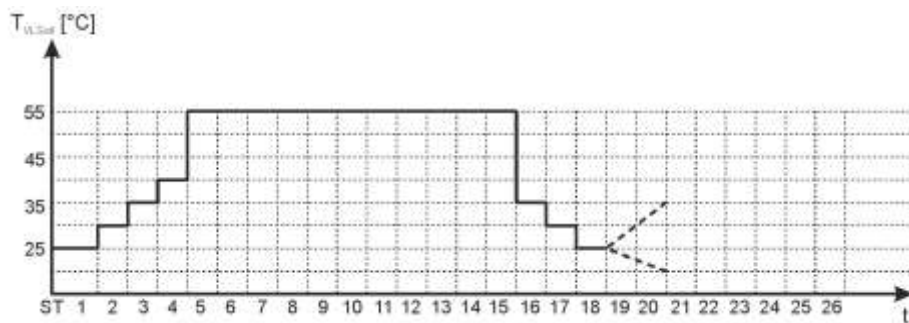
Abb. 71: Zeitlicher Ablauf - Belegreifheizen
