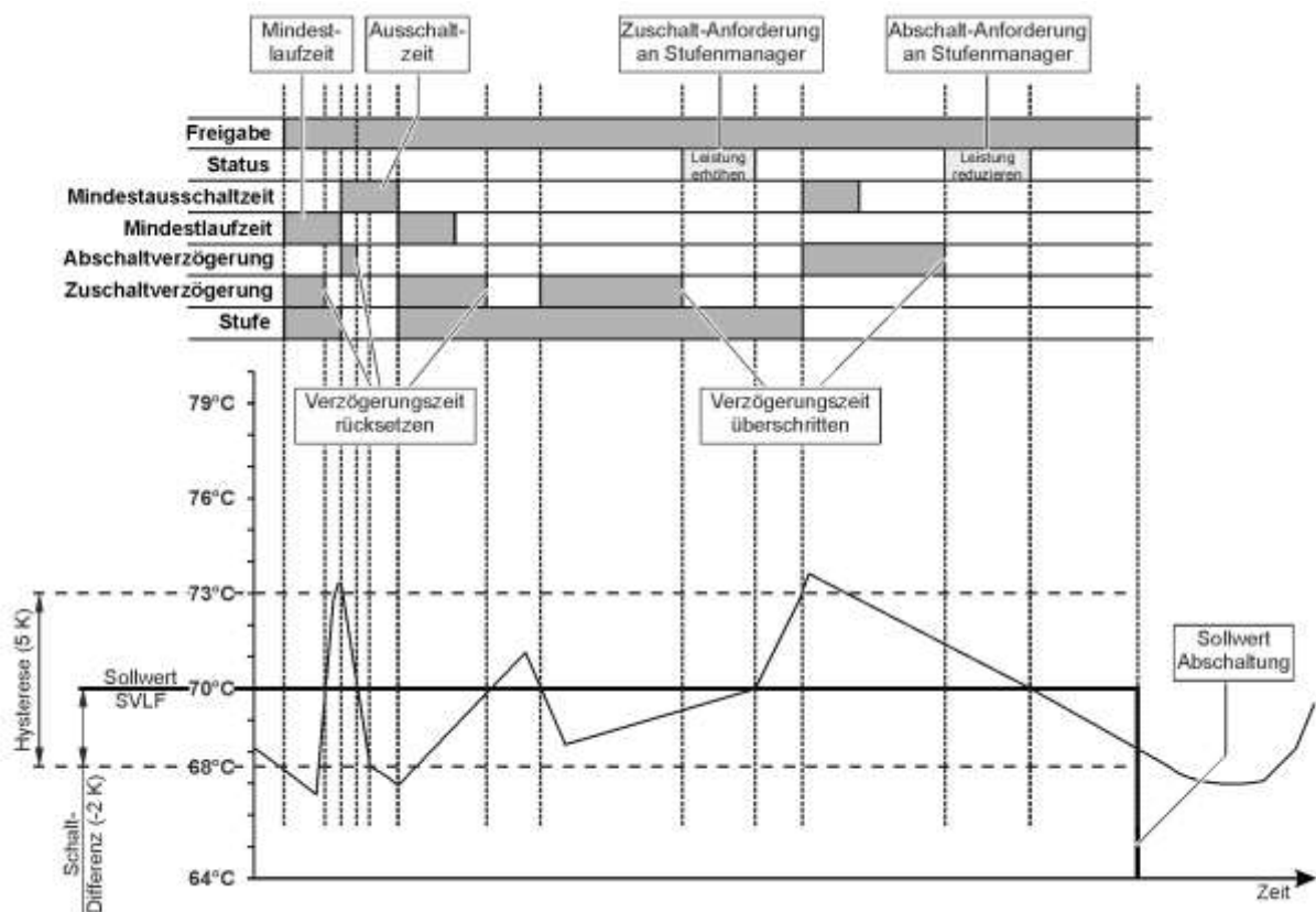
Abb. 54: Stufenmanager (Beispiel)
