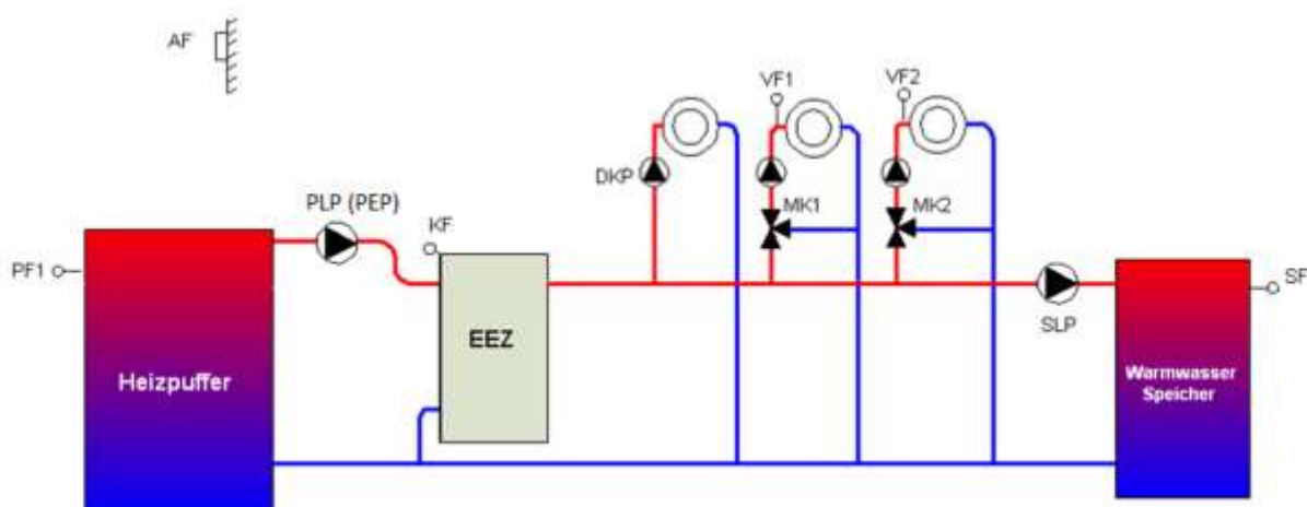
Abb. 82: Pufferentladeregelung 2 auf Wärmeerzeuger
