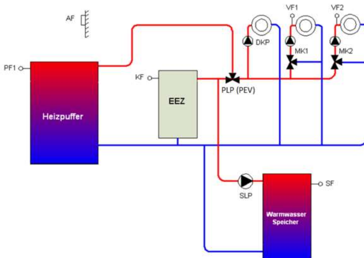
Abb. 81: Pufferentladeregelung auf HK
