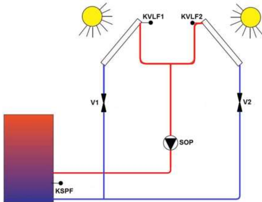
Abb. 84: Solar-Doppelkollektoranlage (Beispiel)
