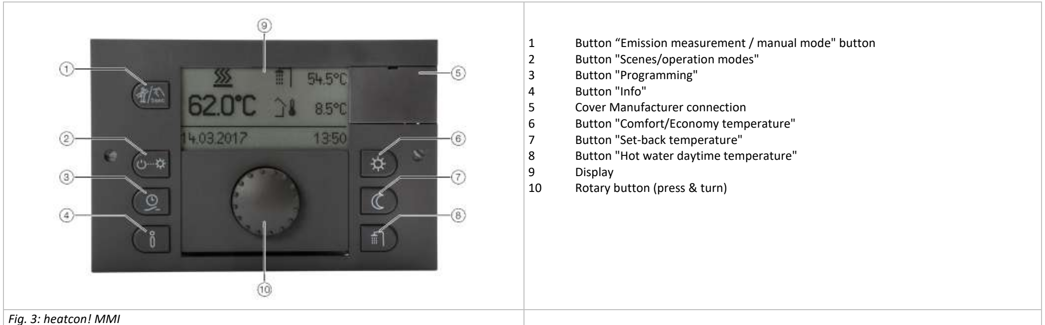
Fig. 3: heatcon! MMI
