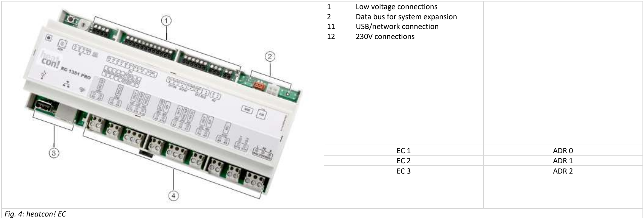
Fig. 4: heatcon! EC
