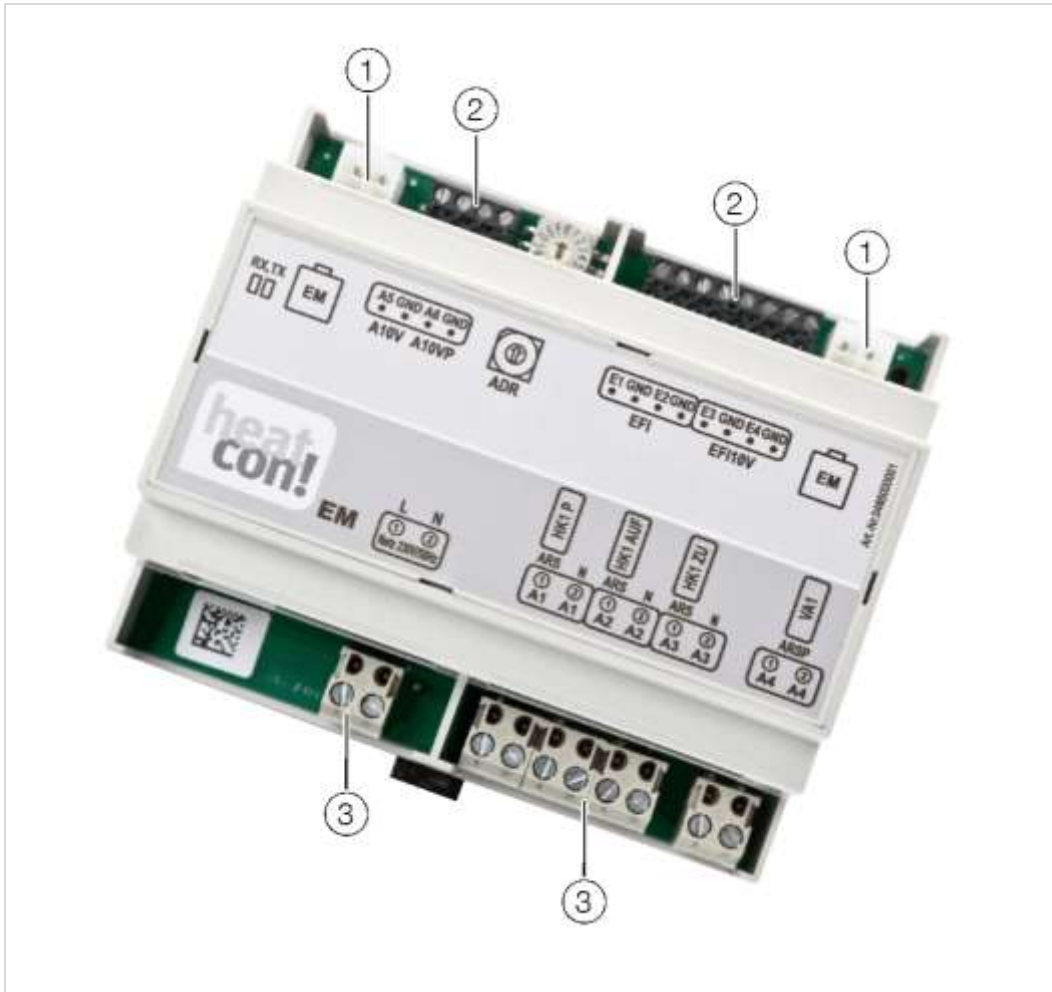
Fig. 5: heatcon! EM 100
