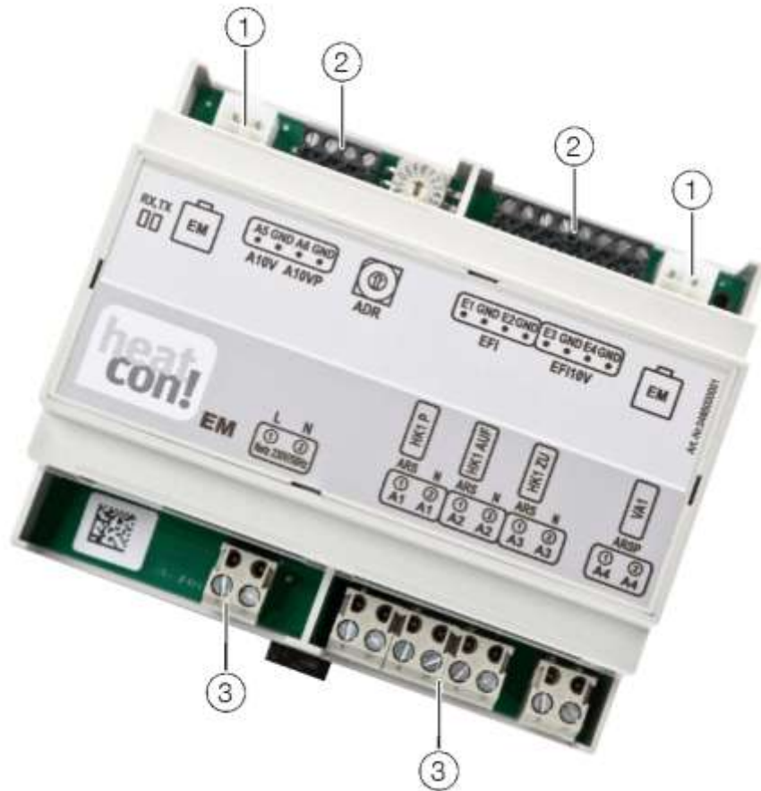
Fig. 5: heatcon! EM 100
