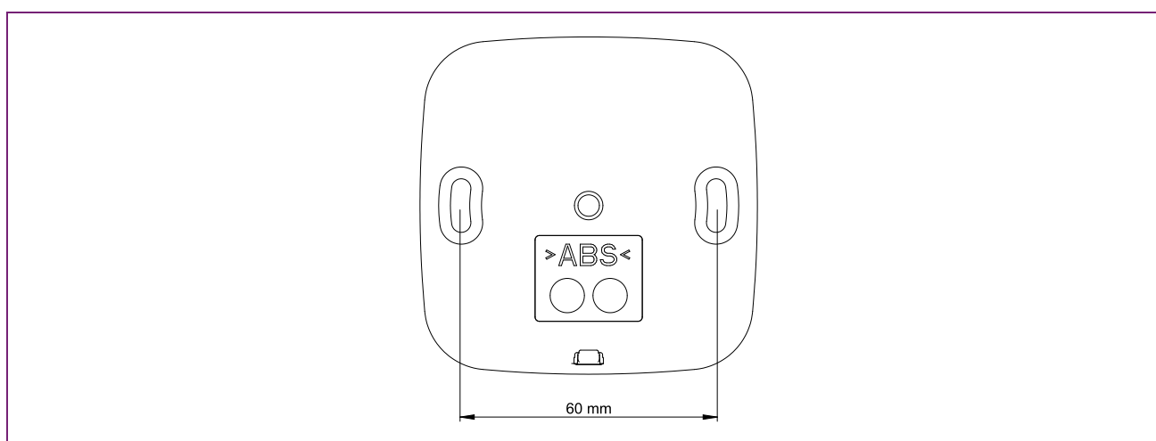
Abb. 1: Bohrbild
