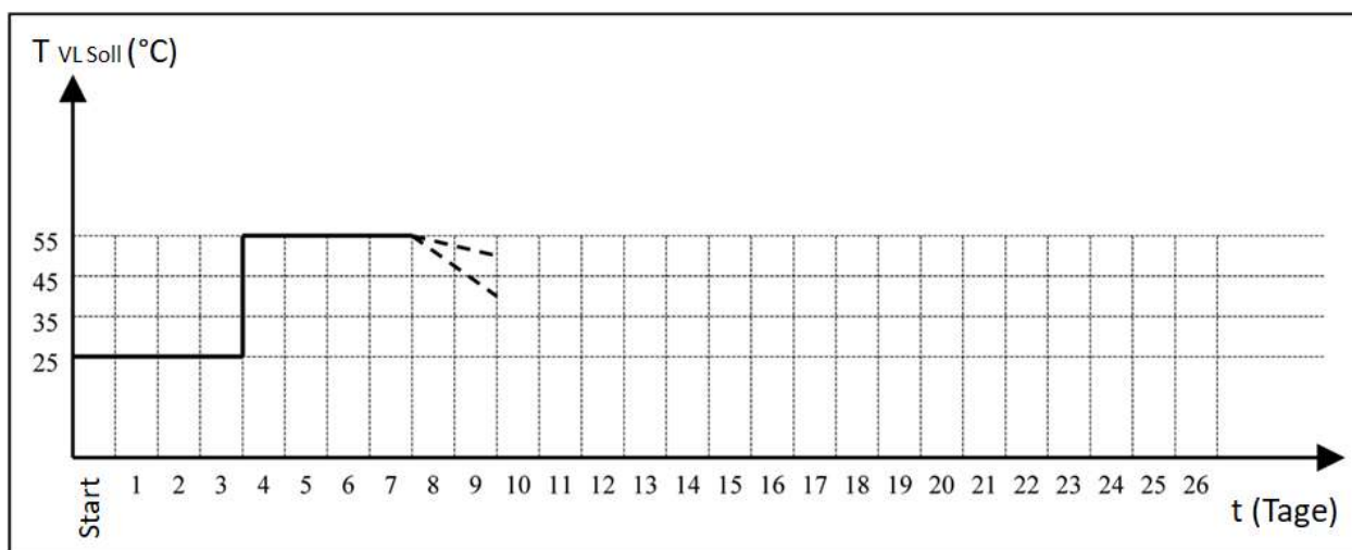
Zeitlicher Ablauf der Estrichfunktion bei Funktionsheizen
