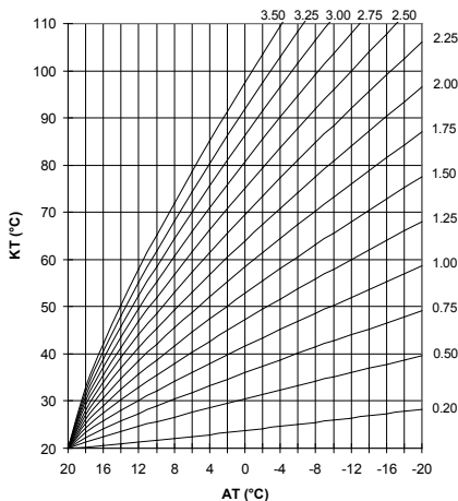
Heizkurvendiagramm
