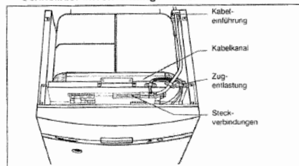
Abb. 4 Steckverbindungen
