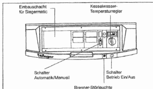
Abb. 2 Bedienelemente
