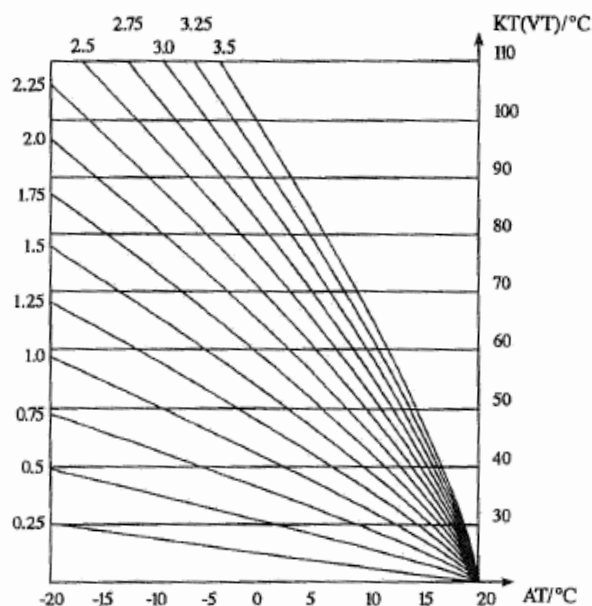
Heizkennlinien-Diagramm
