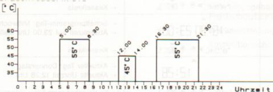
Brauchwasserkreis
