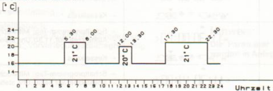
Mischerheizkreis 1
